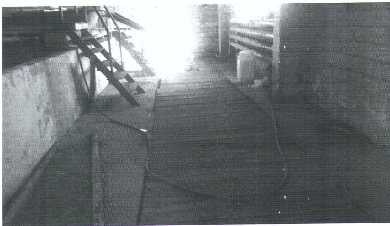
Фото № 7 (Общий вид несанкционированного слива теплоносителя в систему канализации)
